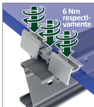
...y apretar todos los tornillos con Torx TX40 (6 Nm).
