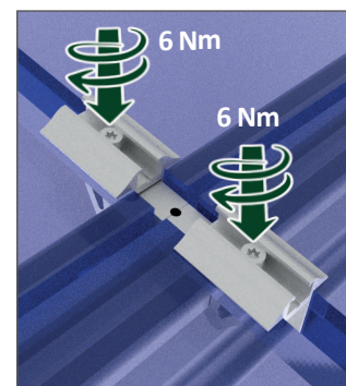
Montaje de la pinza intermedia doble para correa entre los módulos con Torx TX40 (6 Nm)
