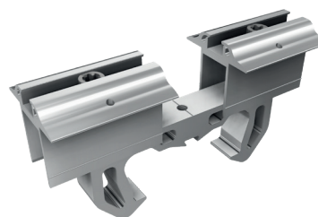
Pinza intermedia doble para correa con puesta a tierra
