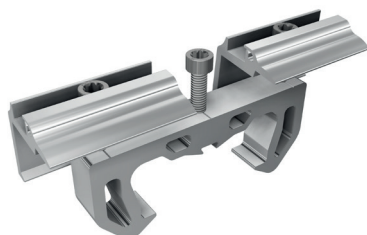
Pinza final doble para correa 30-40 mm
