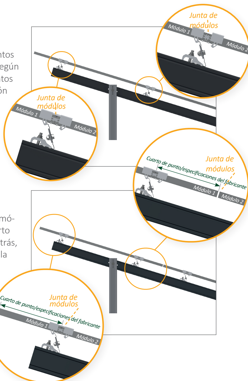
Montaje de la pinza intermedia doble para correa entre los módulos con Torx TX40 (6 Nm)
