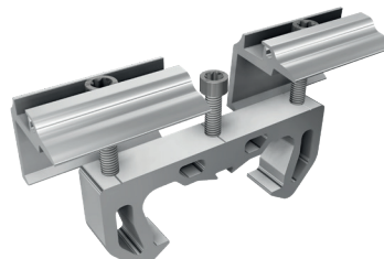
Pinza final doble para correa 41-50 mm
