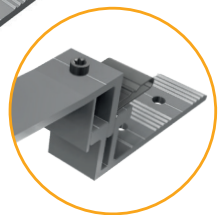
Variante 2: Atornillado a la viga
