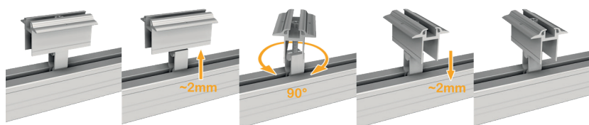
Pinzas finales Vario con clavija de puesta a tierra para una altura del marco de 30 mm - 50 mm
