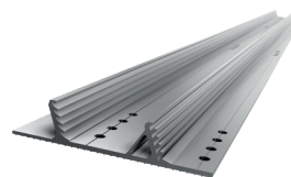
Perfil opcional de cobertura para viga SL Alu-Flex 2000 N.º de artículo 11102-2000
