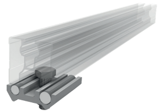
Pinza de protección contra rayos inferior, tornillo hexagonal M10 y tuerca incluidos en el volumen de suministro
