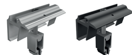
Pinzas finales Vario sin clavija de puesta a tierra para una altura del marco de 30 mm - 50 mm
