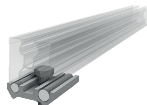
Morsetto parafulmini inferiore, con vite M10 e dado compresi nel materiale in dotazione
